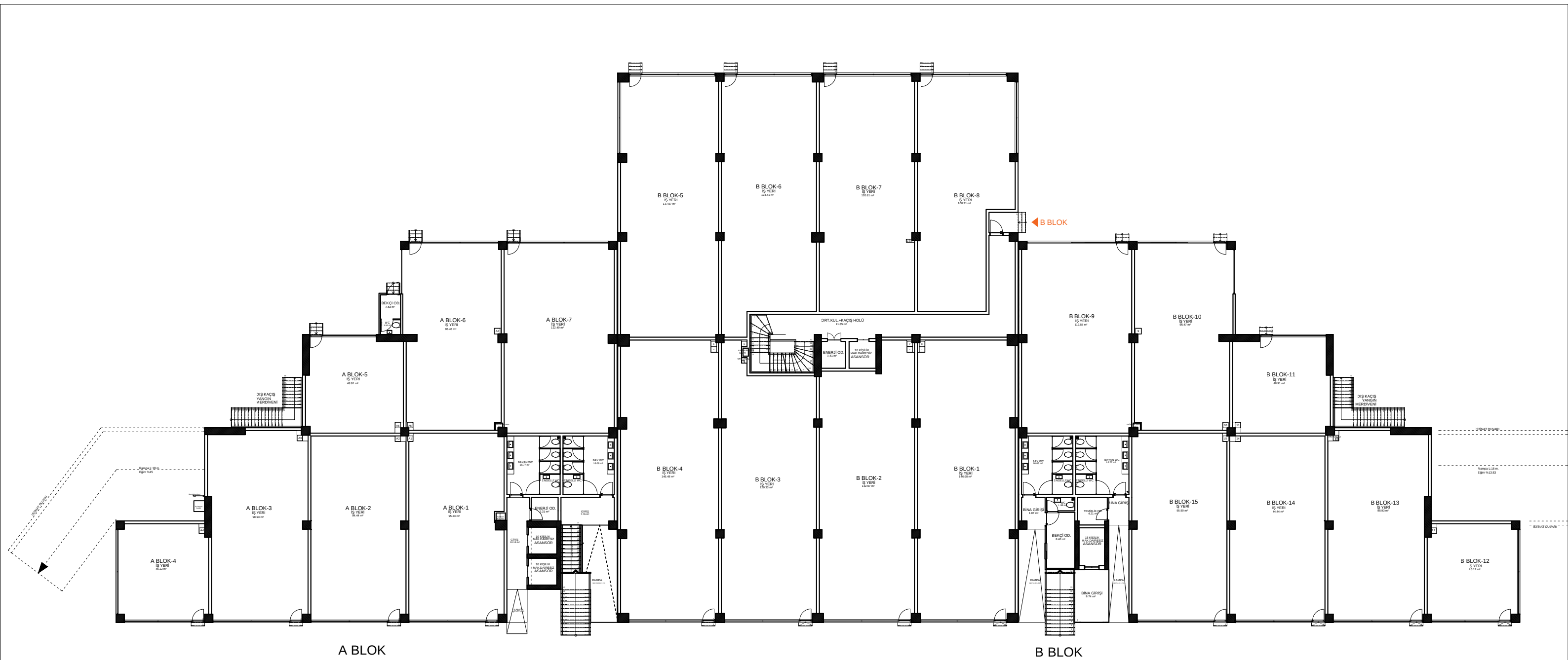
ZEMİN KAT PLANI ÖLÇEK:1/100
